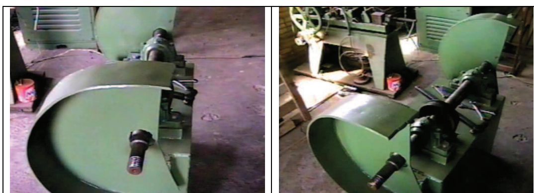
FIGURA 20: Máquina de rebarbeação
