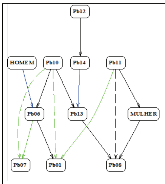
FIGURA 13: Grafo implicativo 2
