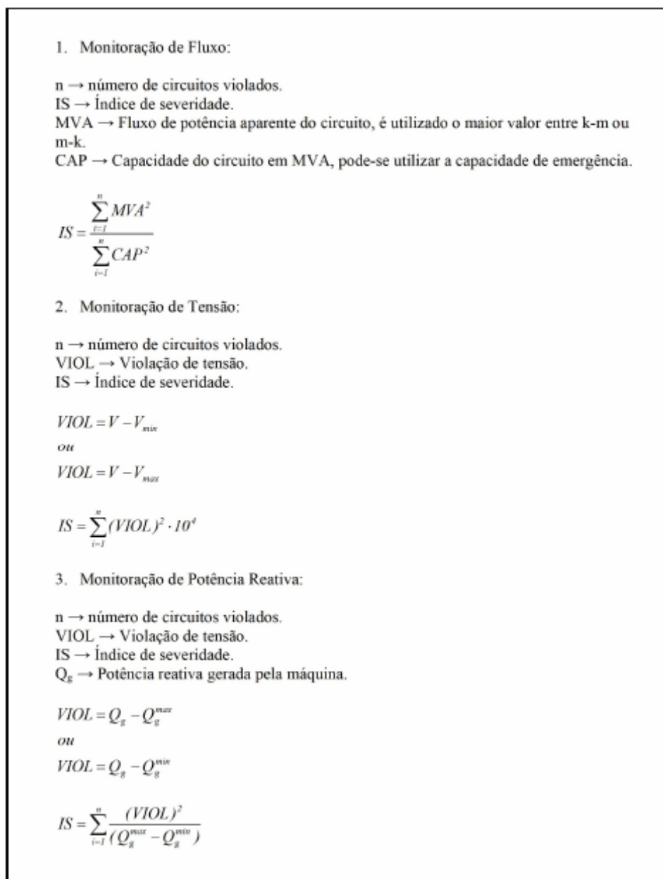
Figura 6.4 – Índices de desempenho utilizados no ANAREDE
