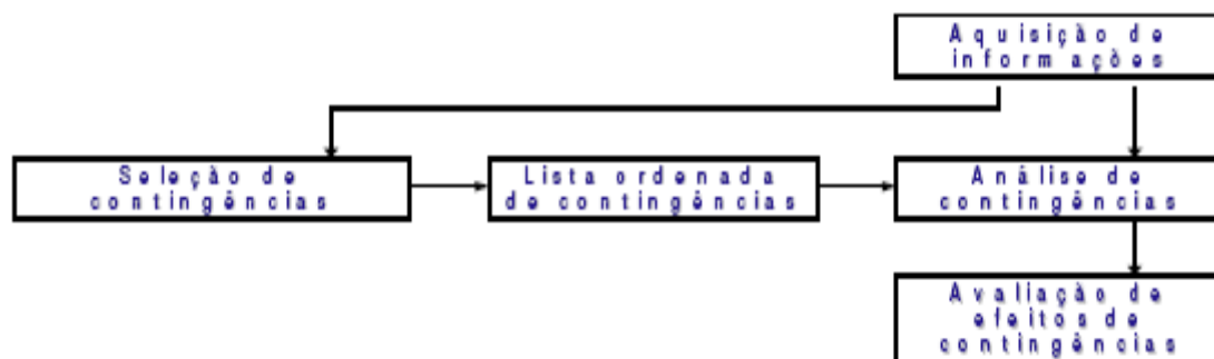
Figura 5.1 – Arquitetura Clássica da Análise de Segurança
