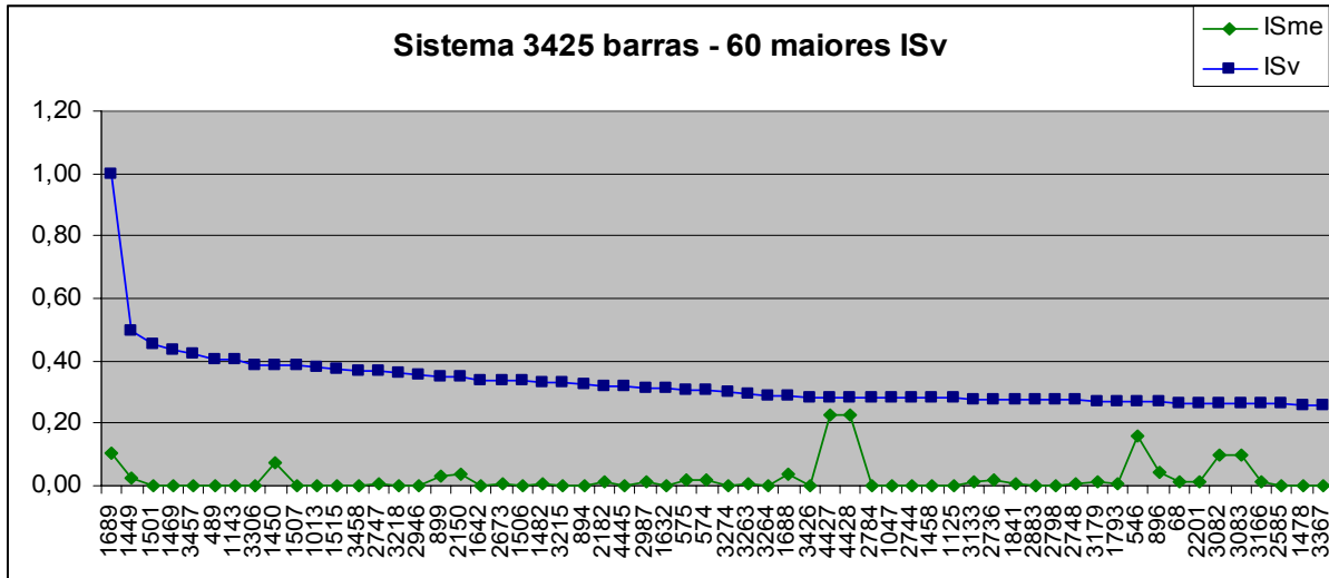
Figura 6.11 – Sistema 3425 – 60 maiores ISv
