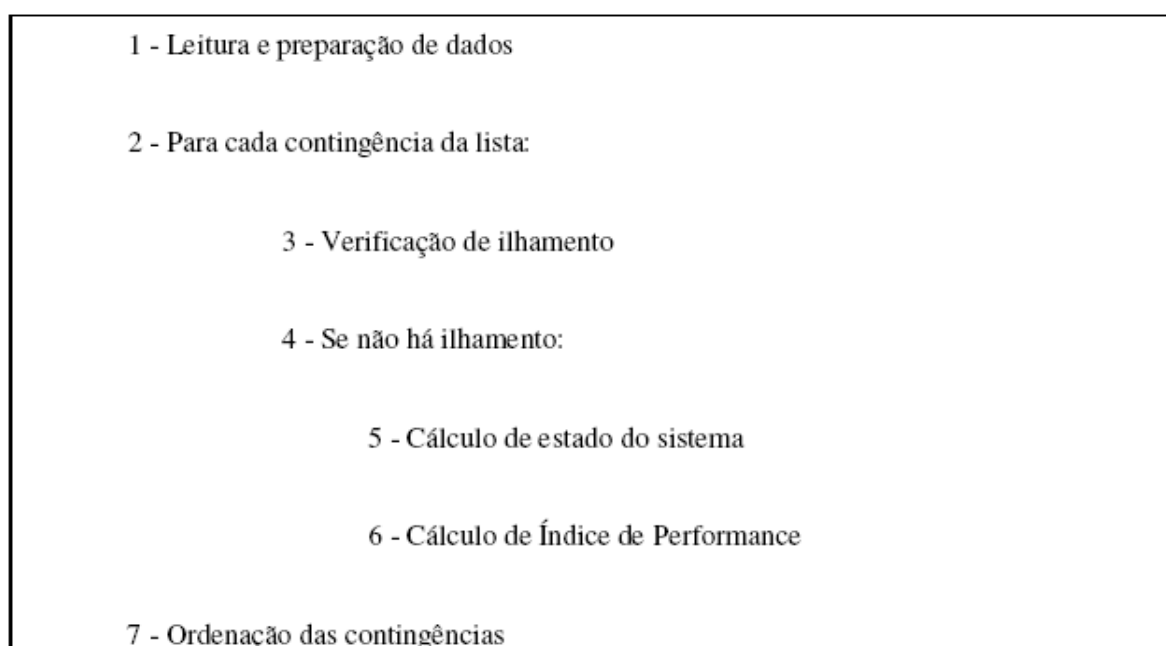
Figura 6.3 – Algoritmo Geral
