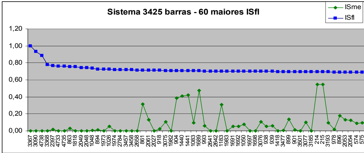
Figura 6.10 – Sistema 3425 – 60 maiores ISfl
