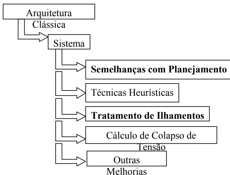
Figura 6.1 - Módulos desenvolvidos
