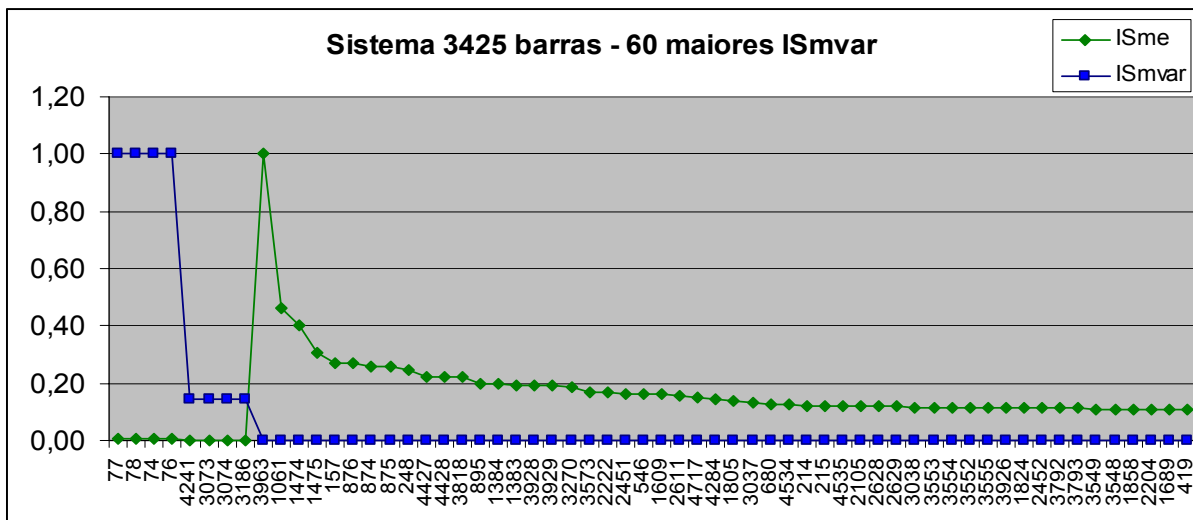
Figura 6.12 – Sistema 3425 – 60 maiores ISmvar
