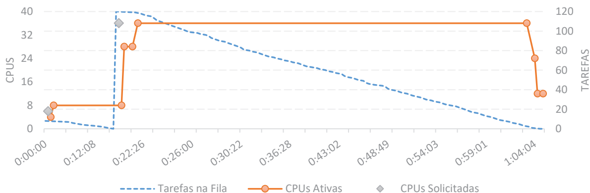
Figura 45 – Comportamento de elasticidade para uma execução do arquivo 12-stamatakis-59 no cenário C_{c36} .
