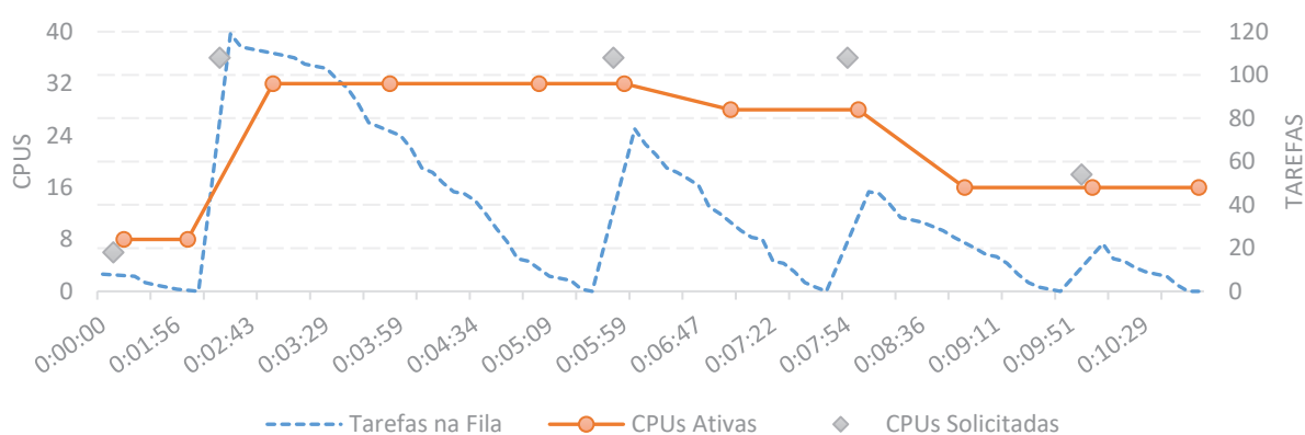
Figura 42 – Comportamento de elasticidade para uma execução do arquivo 08-HIV_vpu.ref2 no cenário C_{c36} .
