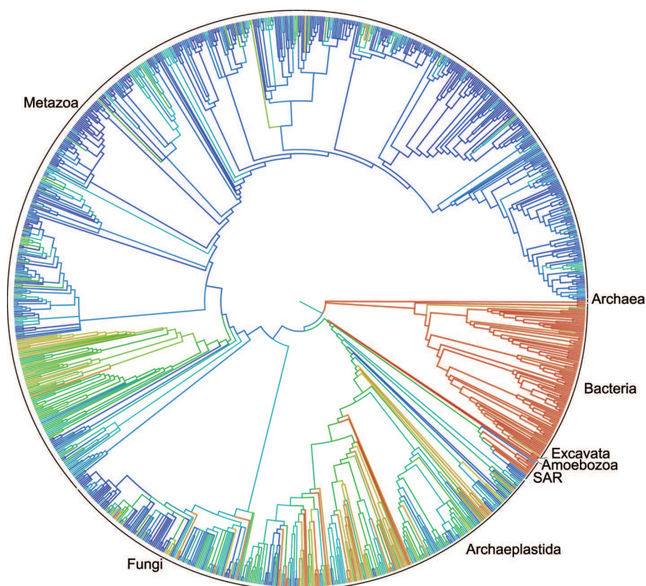
Figura 2 – Representação gráfica de uma árvore filogenética em uma tentativa de reconstruir a hipotética Árvore da Vida até o ancestral universal.
