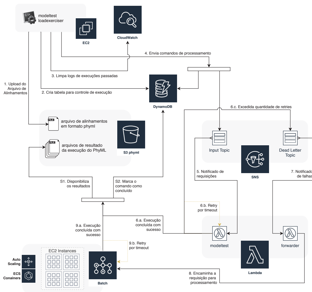
Figura 25 – Diagrama da arquitetura adotada no desenvolvimento do protótipo He-lastic, descrevendo as etapas do fluxo de execução, assim como os serviços utilizados, representando a implementação do ambiente de computação em nuvem retratado na arquitetura do modelo (Figura 15).
