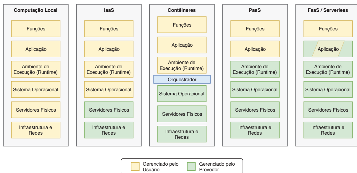
Figura 6 – Diagrama representando a divisão de responsabilidades sobre as diversas camadas que compõem um ambiente computacional contrastando ambientes locais com diferentes modelos de serviço habilitados pela computação em nuvem (IaaS, PaaS, Contêineres, e FaaS).
