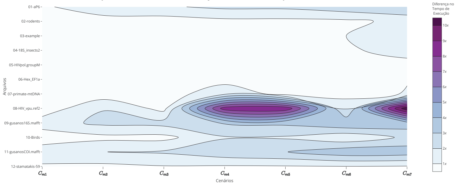
Figura 47 – Mapa de calor da diferença nos tempos de execução entre os cenários de avaliação do modelo He-lastic com FaaS e Orquestração de Contêineres versus os cenários do jModelTest, onde cores mais fortes representam maiores diferenças.
